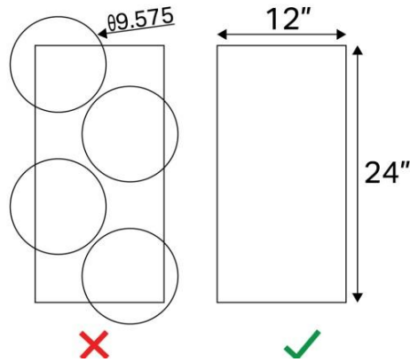
图 R19-1：自制塑料件须可容纳于单块 12" × 24" 的塑料板内。
