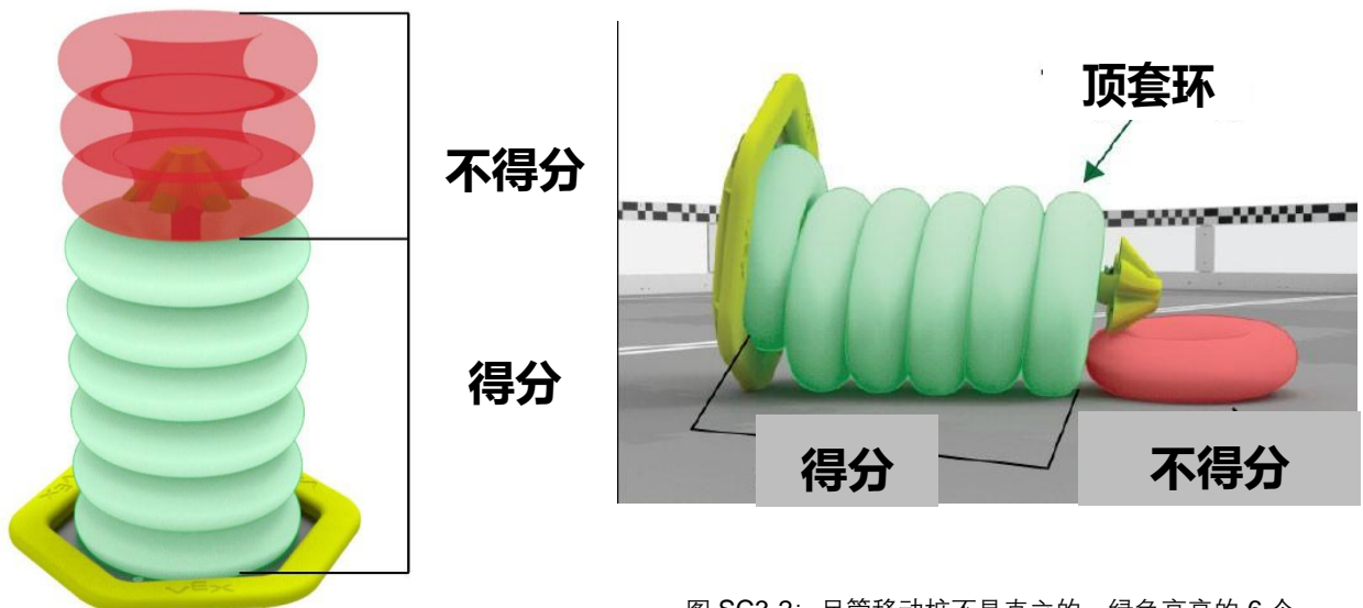
图 SC3-2：尽管移动桩不是直立的，绿色高亮的 6 个套环仍记分，因为他们符合上述所有标准。红色高亮套环不记分，因为它没有“环绕”尖桩。
