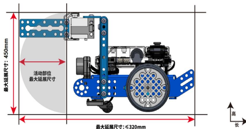
图 5.1-1 最大延伸尺寸-侧视图
