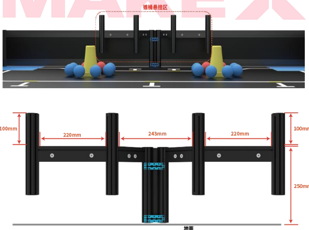
图 4.2-5 锥桶悬挂区示意图
