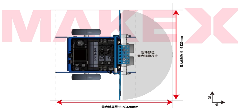
图 5.1-2 最大延伸尺寸-俯视图
