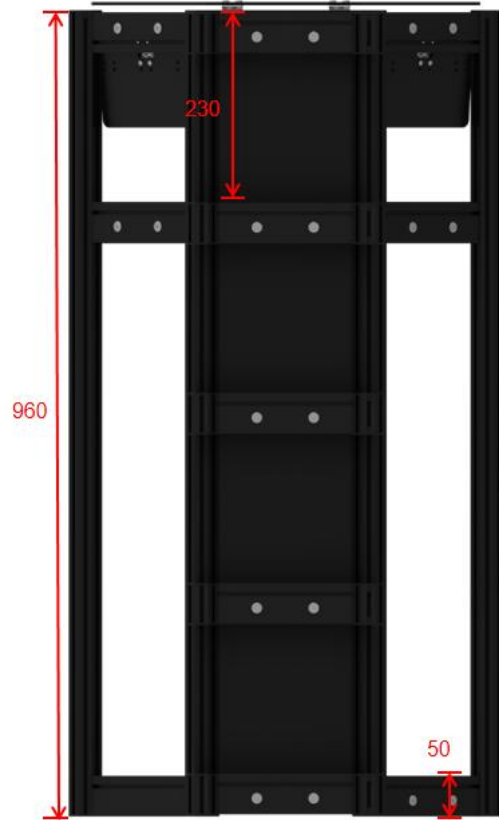
图 4.2-17 中央资源岛示意图（正视图）
